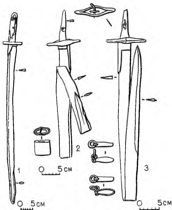
Рис. 19. Сабли и железные детали ножен аскизской культуры 1 — грот I скалы Узун хая (начало XI в.); 2 — курган 12 у д. Черновой (палаш? — конец XII — начало XIII в.); 3 — курган 1 могильника Самохвал II (XIII в.)
