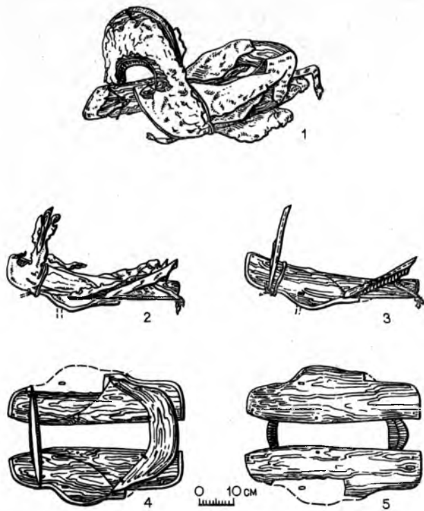
Рис. 18. Седло из погребения в гроте I скалы Узун хая (Хакасия, начало XI в.). Общий вид (дерево, шкура овцы, кожаные ремни) и детали конструкции
