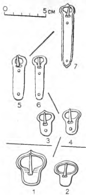
Рис. 17. Основные тенденции развития неподвижнощитковых пряжек IX—XII вв.
