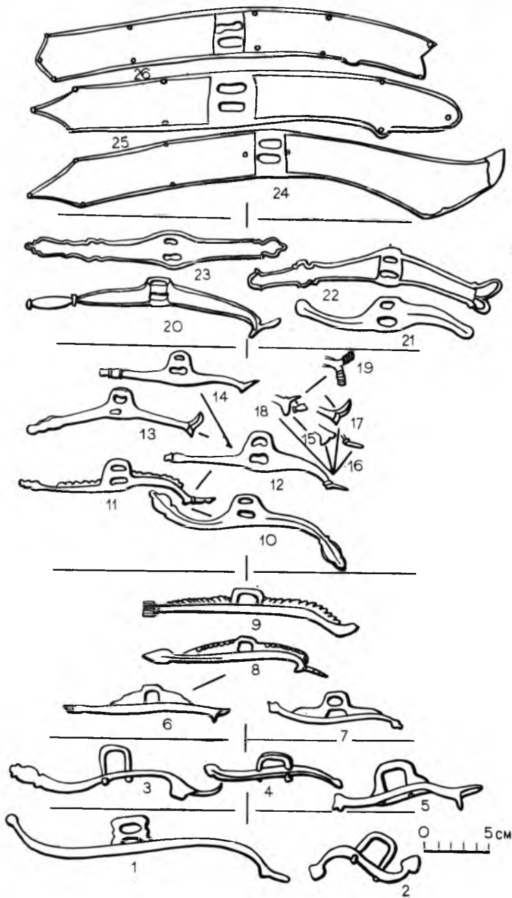
Рис. 7. Типологическая последовательность развития вертикальных псалиев в VIII—XIV вв. (культуры чаатас, тюхтятская и аскизская)
