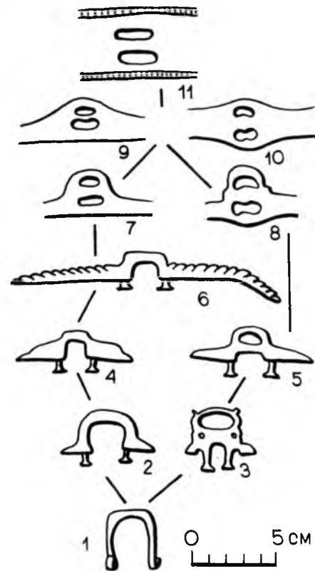
Рис. 6. Типологическая последовательность развития скоб для нащечного ремня узды у псалиев в условиях культур чаатас, тяхтатской в аскизской (VII—XIV вв.)
