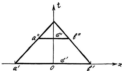
Рис. 2. Если даны только начальные данные на \sigma'(a'b') и неизвестны граничные данные, то область \sigma'' , в которой известно поле \varphi , сокращается со скоростью света c , и при t = a'b'/c \sigma'' = 0 !
