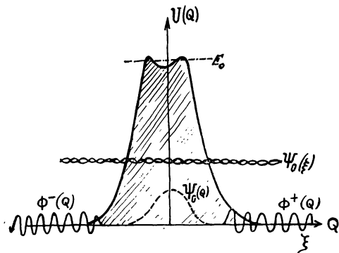
Рис. 10. Здесь изображена потенциальная энергия U(Q) тяжелого шарика. E_0 — исходное состояние. На этом же графике введены волновые функции \Psi_0(Q) , \Psi_0^\mp(Q) и \Psi_0(\xi)
