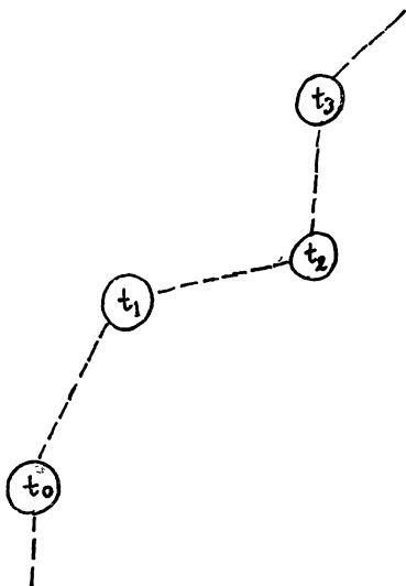
Рис. 12. Траектория микрочастицы как последовательность макроскопических событий: каждый кружок означает макроскопические явления, вызванные микрочастицей. Например, кружок может означать пузырьки пара в пузырьковой камере
