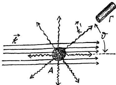
Рис. 6. Первичная волна \vec{k} рассеивается на микросистеме А, рассеянная волна \vec{k}' показана волнистыми линиями. Г — счетчик частиц, рассеянных на угол \varphi
