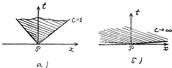
Рис. 5. Область влияния событий в точке P на события при t > 0 : а) в релятивистской теории, б) в классической
