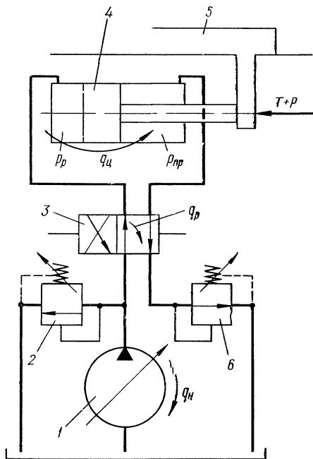
Рис. 28. Принципиальная схема объемного способа регулирования скорости
