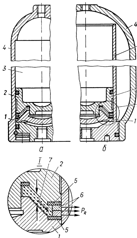
Рис. 103 Аккумулятор фирмы «Ате»: a — первый вариант конструкции; 1 — нижняя часть поршня; 2 — верхняя часть поршня; 3 — газовая среда; 4 — баллон-цилиндр; б — второй вариант конструкции; 1 — нижняя часть поршня; 2 — верхняя часть поршня; 3 — направляющая гильза; 4 — баллон; 5 — упругое кольцо; 6 — уплотнительное кольцо; 7 — уплотнение из эластичной резины
