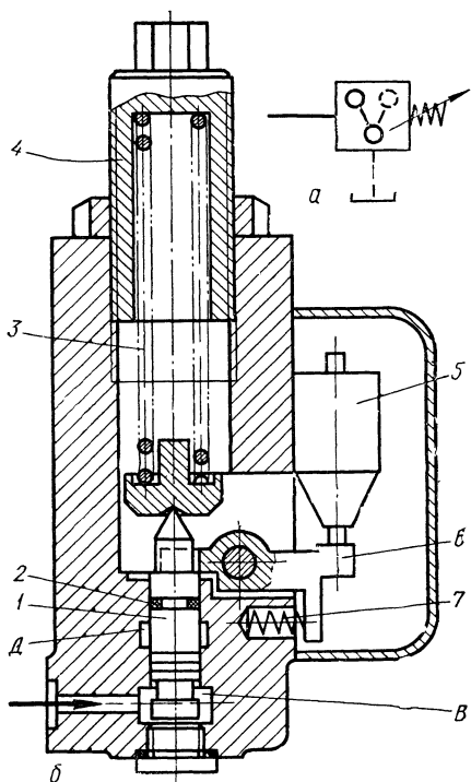
Рис. 9. Реле давления типа ПГ62-11:
