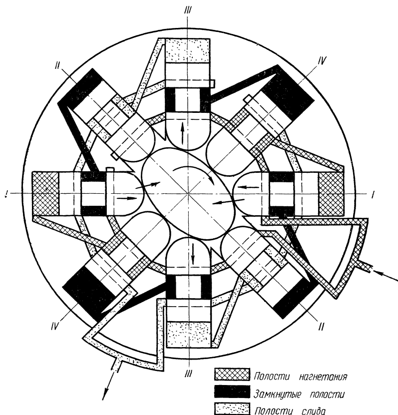
Рис. 27. Гидромотор Acra Drive фирмы «Cincinnati»
