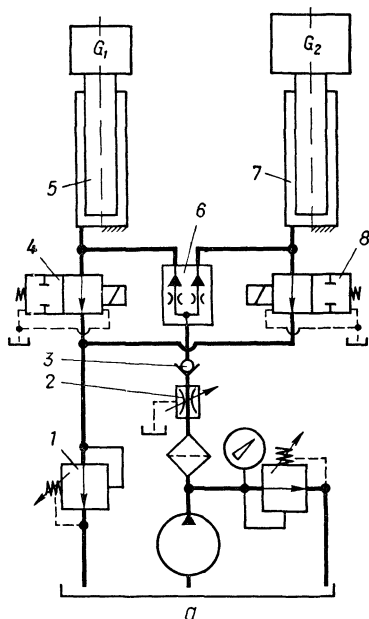
Рис. 73. Гидросистемы, обеспечивающие синхронную работу цилиндров одностороннего действия
