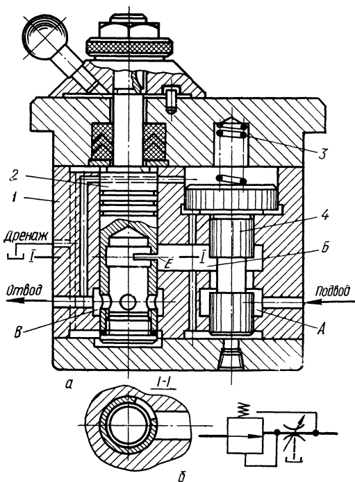
Рис. 10. Дроссель с регулятором типа Г55-2:
