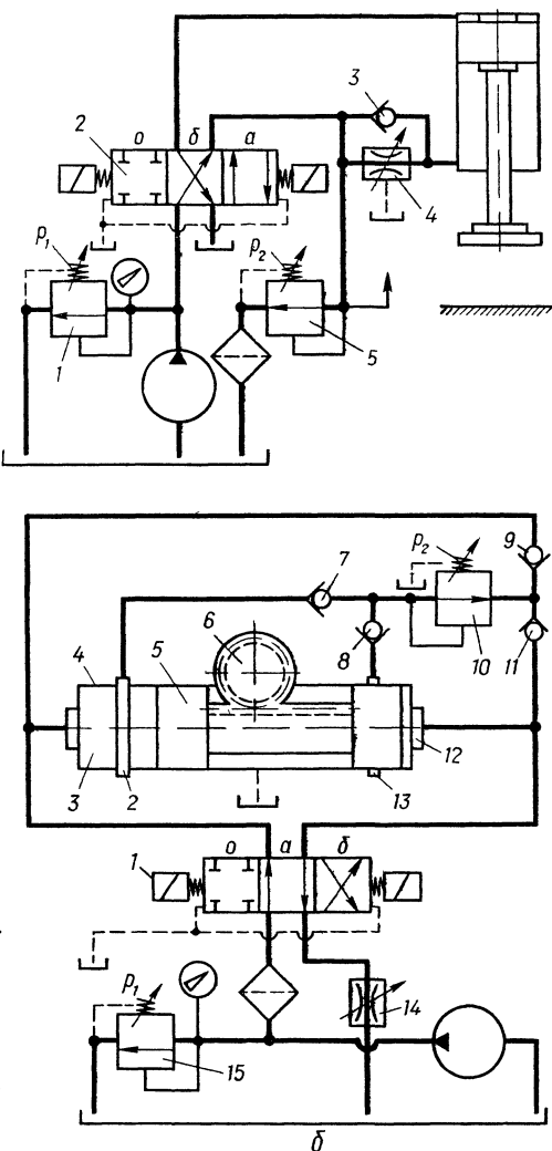
Рис. 54 Гидравлические системы, обеспечивающие частичную разгрузку насоса:
