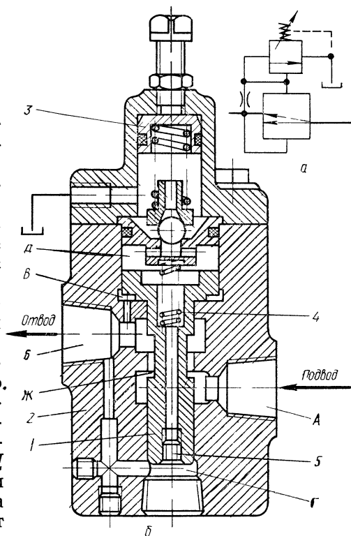
Рис. 8. Клапан редукционный с регулятором типа Г57:
