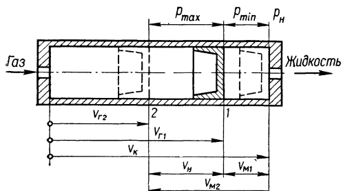
Рис. 107. Схема к выбору параметров газогидравлического аккумулятора
