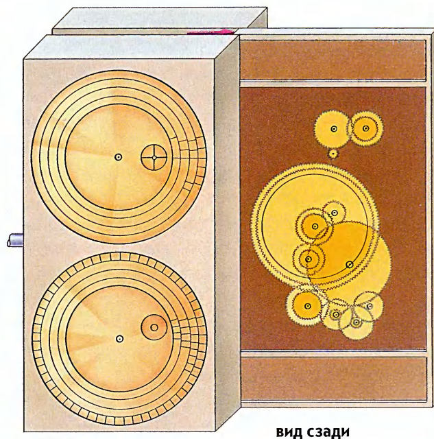
Схема механизма, своего рода «астрономического компьютера», с острова Антикитеры. Его возраст — почти две тысячи лет.
