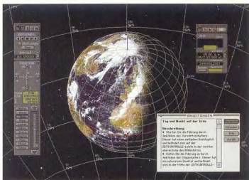
День и ночь на Земле, вращающейся вокруг Солнца. Кадр из записанного на компакт-диске курса астрономии, в котором объясняются многие космические явления, показанные в фильме со спецэффектами.
