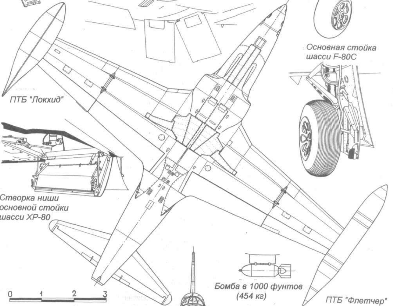
Нижняя часть фюзеляжа F-80C
