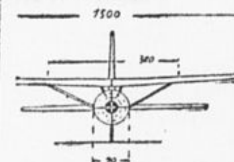
Рис. 2. Средняя часть планера спереди.
