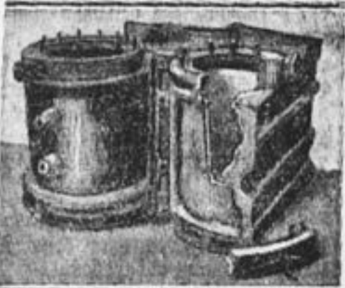
Лопнувший паровозный цилиндр до сварки.
