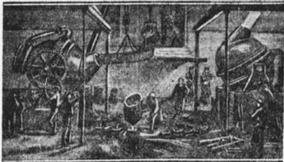
НАЛЕВО—«груша Бессемера» в момент наполнения ее чугуном. НАПРАВО—во время выжигания в ней углерода посредством продувания снизу воздуха.
