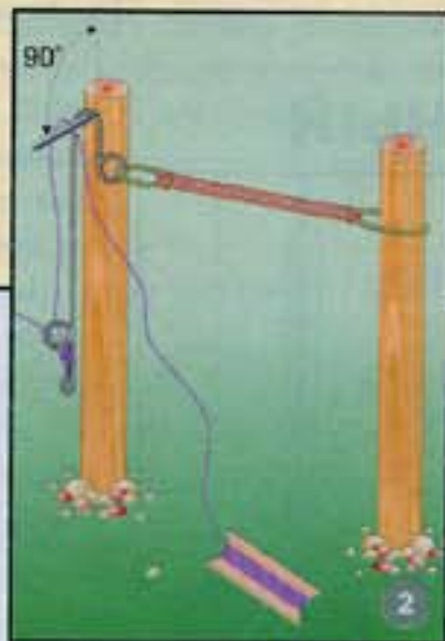
2. Установка «Кнута» на берегу, на деревянных кольшках.
