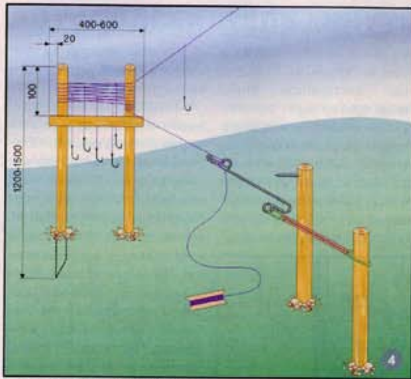
4. Стойка для ловли с «Кнутом».
