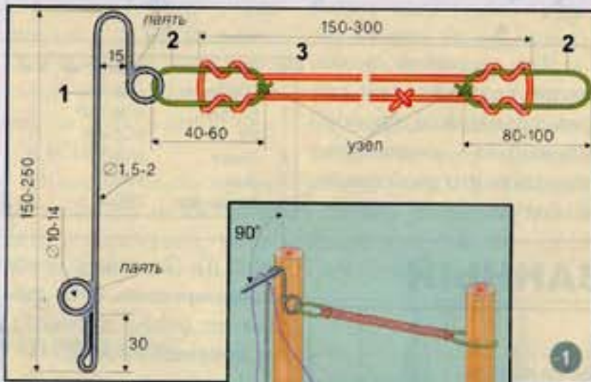
1. Схема автоподсекателя «Кнут»: 1 – сторожок; 2 – петли; 3 – пружина из резины.
