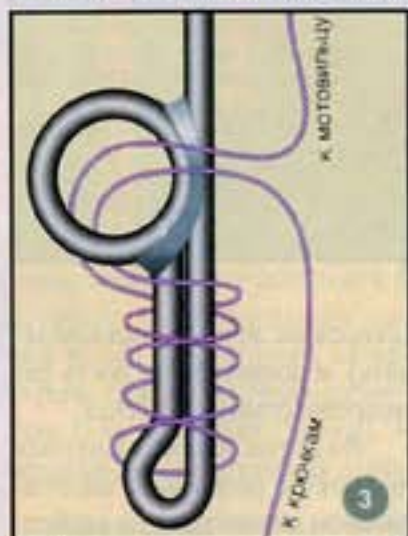
3. Крепление лески к автоподсекателю с помощью петли.
