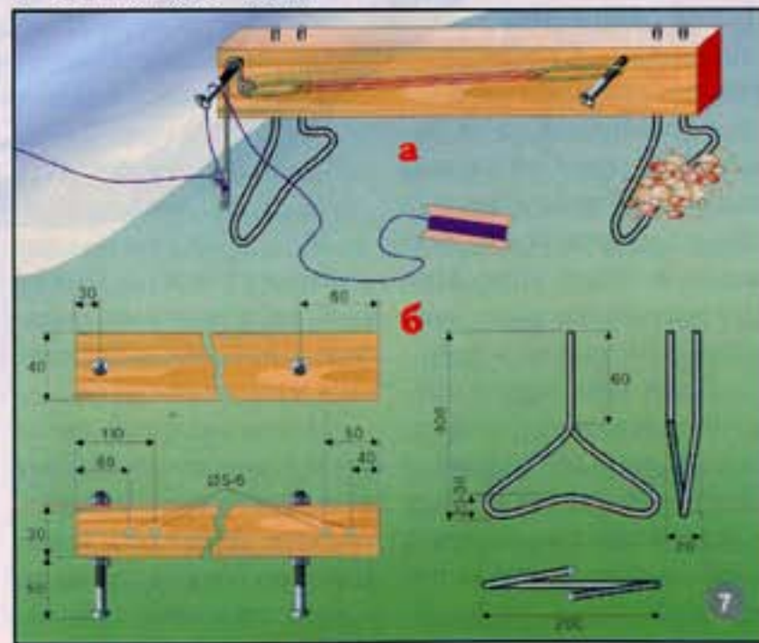
7. Опора для крепления «Кнута» со съемными ножками: а – внешний вид; б – схема.
