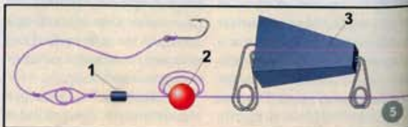
5. Огрузка для ловли с «Кнутом»: 1 – грузильце; 2 – стопор; 3 – скользящее грузило.
