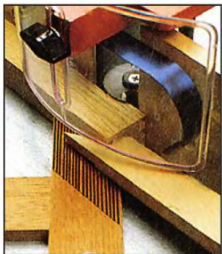
Вспомогательный упор для прижима надёжно удерживает последний.
