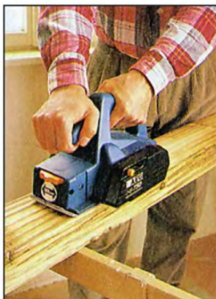
Рустикальная обработка пласти заготовки электрорубанком, оснащённым специальными профильными ножами.
