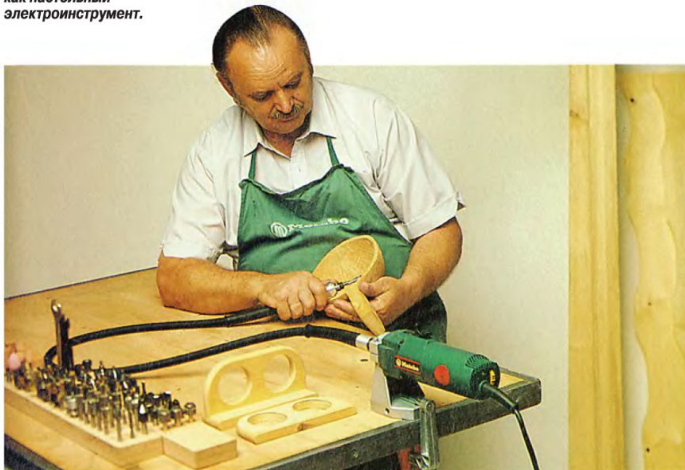
Гибкий вал установлен на электропривод фрезерной машинки.
