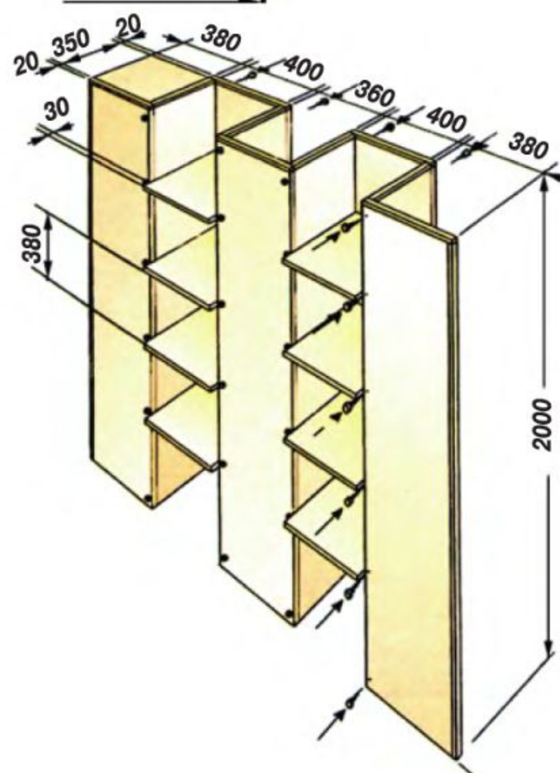
Рис. 2. Размеры самодельного стеллажа — 2000х2000х420 мм. Материал для его изготовления — ДСП толщиной 19 мм. Стенки стеллажа соединены друг с другом саморезами. Кромки деталей стеллажа облицованы декоративными накладками. Полки раскраивают так, чтобы они спереди несколько выступали за пределы стенок. К стенкам их крепят также саморезами. С тыльной стороны стеллажа полки устанавливают только в его средней части. Собранный стеллаж покрывают прозрачным лаком.
