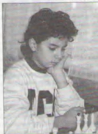
№ 60 Защита Пирца-Уфимцева
