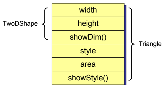
Рис. 11.1. Схематическое представление класса Triangle
