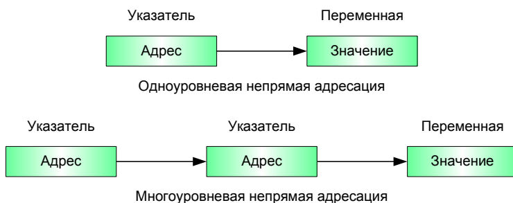
Рис. 18.1. Одноуровневая и многоуровневая непрямая адресация
