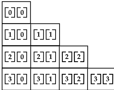
Рис. 3.2. Двумерный массив с различными размерами второго измерения
