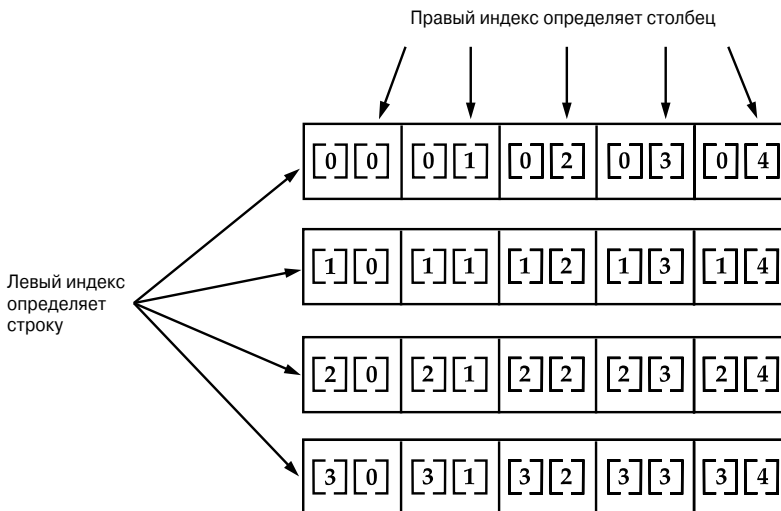
Рис. 3.1. Логическое представление двумерного массива 4 \times 5
