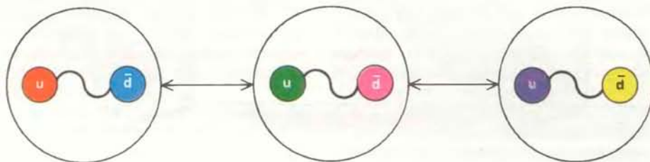
\pi^+ -МЕЗОН
