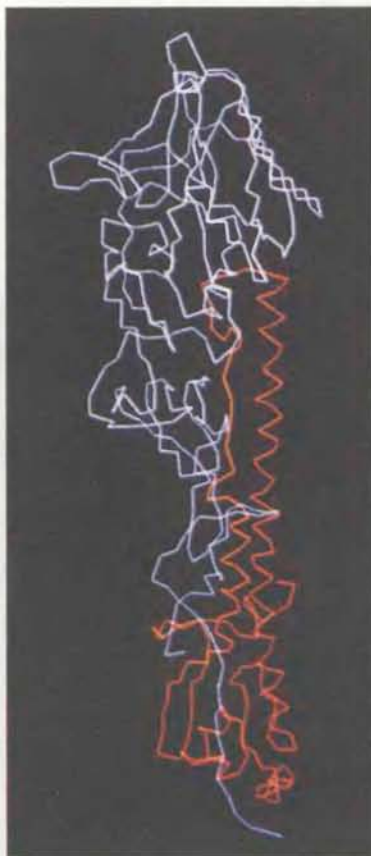
МОЛЕКУЛА ГЕМАГГЛЮТИНИНА вируса гриппа состоит из двух полипептидных цепей: HA 1 (фиолетовая) и HA 2 (оранжевая). Трехмерная модель молекулы (слева) построена по данным рентгеноструктурного анализа, полученным А. Уилсоном и Д. Уили (Гарвардский университет) и Дж. Скехелом (Национальный институт медицинских исследований, Лондон); показан лишь остов белка. Тример гемогглютинина (справа) содержит три цепи HA 1 и три цепи HA 2 . Тримеры образуют шипы на сферической оболочке вирусной частицы.
