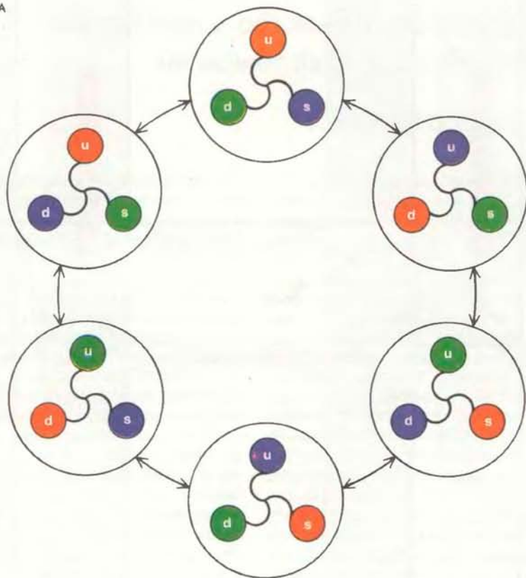
\Lambda -ЧАСТИЦА
