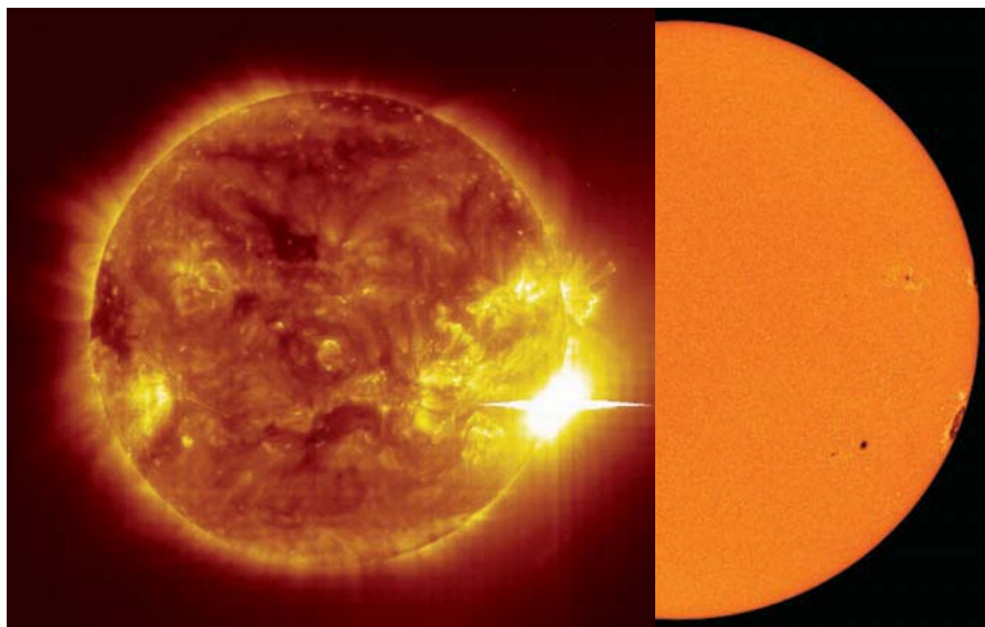
В результате рекордно сильной вспышки, произошедшей 4 ноября 2003 г. вблизи солнечного края, датчик ультрафиолетового телескопа на спутнике SOHO ( Solar and Heliospheric Observatory — Солнечная и гелиосферная обсерватория) зашкалило. В результате осталась ложная горизонтальная линия (слева). Как и в других подобных случаях, рядом расположено солнечное пятно, т.е. область интенсивного магнитного поля (справа)
