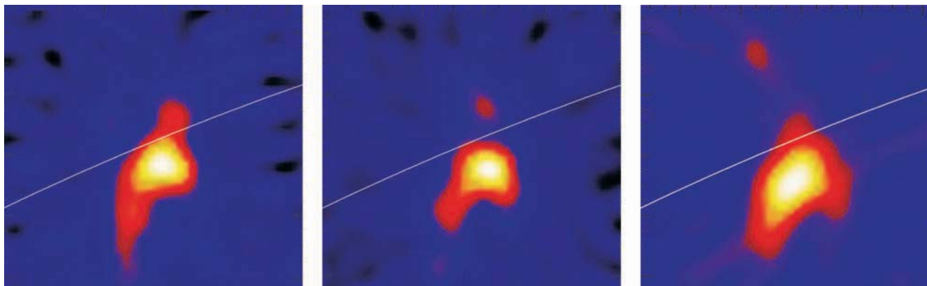
На серии рентгеновских снимков, полученных RHESSI , видна вспышка 15 апреля 2002 г., сопровождавшаяся выбросом корональной массы. Источник рентгеновского излучения появился как красное вздутие над основной петлей горячего газа ( слева ) и над видимым краем Солнца ( белая линия ). Он несколько минут оставался неподвижным, пока вершина петли опускалась ( в центре ), но затем был выброшен в пространство ( справа ). Все это подтверждает предположение, согласно которому за вспышку и выброс корональной массы ответственно пересоединение силовых линий на вершине магнитных петель. Мы действительно наблюдаем то, что можно ожидать в рамках данного сценария: после пере замыкания магнитного поля у вершины петлей половина вновь сформированных силовых линий должна переместиться вниз, а другая часть — сдвинуться вверх, вызывая выброс корональной массы
