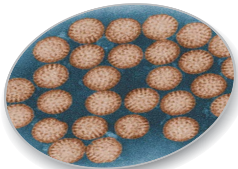
Под электронным микроскопом видны маленькие колесики — это и есть ротавирусные частицы (отсюда и их название: rota в переводе с латинского означает «колесо»). Для наглядности они слегка окрашены
