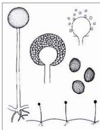
Фотография и схематическое изображение мицелия, спорангиев и спорангиев Rhizopus
