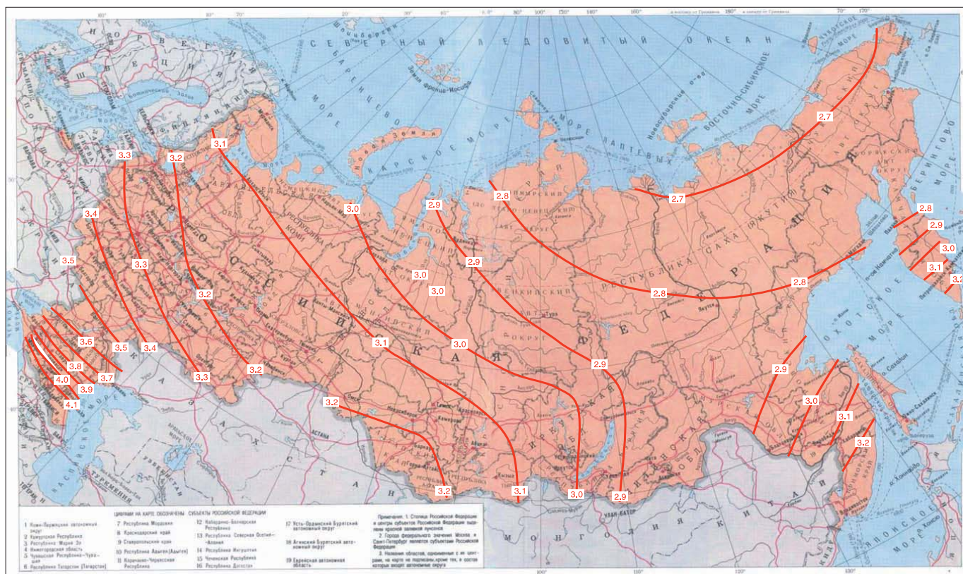
Районирование территории России по эффективности использования низкотенциальной тепловой энергии поверхностных слоев земли
