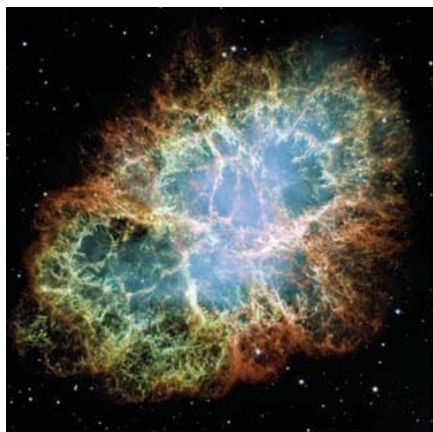
Крабовидная туманность — газовый остаток сверхновой с коллапсом ядра, взрыв которой наблюдался в 1054 г. В центре — нейтронная звезда (указана стрелкой), выбрасывающая частицы, заставляющие газ светиться (голубой). Внешние волокна в основном состоят из водорода и гелия разрушенной массивной звезды
