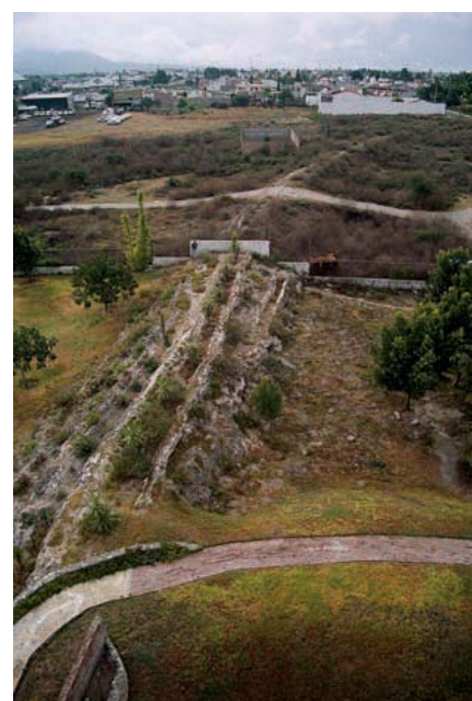
Три параллельных текоатля (справа): меньшие из них представляют собой боковые ветви, которые вели к соседним полям. Основное русло доходит до современного центра города Теуакан, где при прокладке современных улиц (вверху) каналы были частично разрушены
