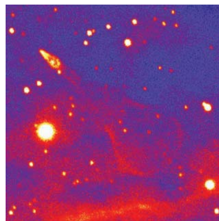
Туманность гитара — это ударная волна, расходящаяся за нейтронной звездой (у стрелки), которая несется сквозь газ со скоростью 1600 км/с. Чтобы сообщить звезде такую скорость, взрыв должен быть несимметричным
