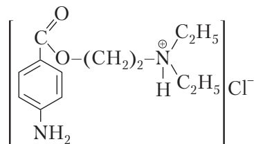
новокаина гидрохлорид
