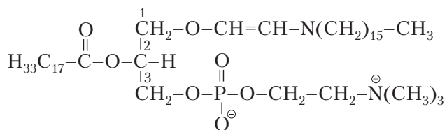
1-О-(октадецен-1-ил)-2-олеилфосфатидилхолин
