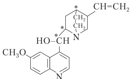
хинин
