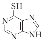
6-меркаптопурин
