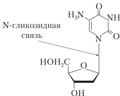
тимидин
