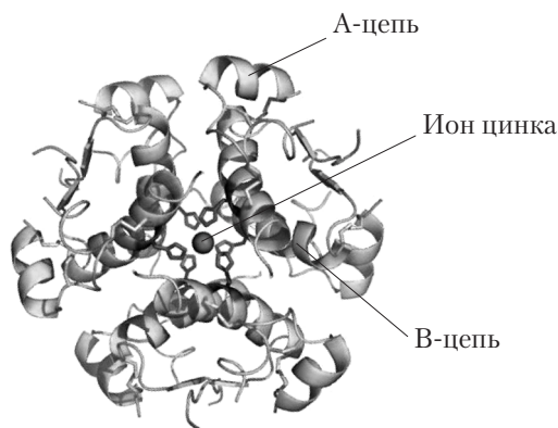
Рис. 15.3. Пространственная структура гексамера инсулина (вид сверху)
