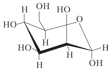
\alpha - D -маннопираноза (устойчивая конформация)
