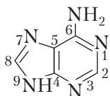
аденин (6-аминопурин)
