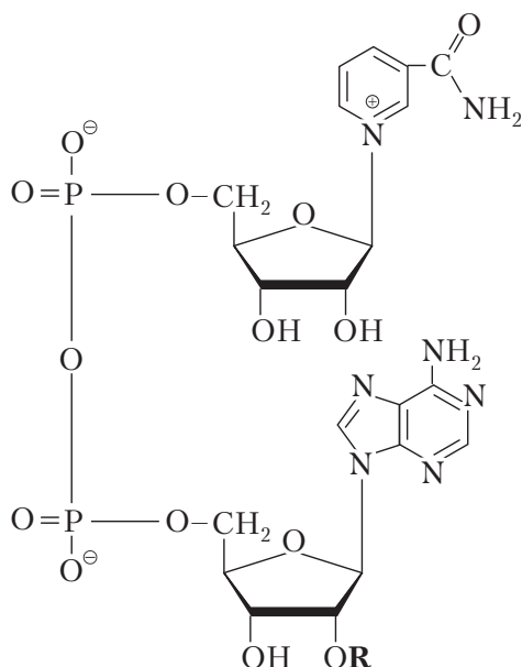
Рис. 16.2. Строение никотинамидадениндинуклеотида: R = \text{H} - \text{НАД}^+ ; R = \text{PO}_3^{2-} - \text{НАДФ}^+
