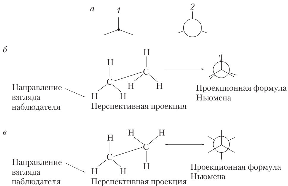
Рис. 3.5. Изображение в проекционных формулах Ньюмена:
