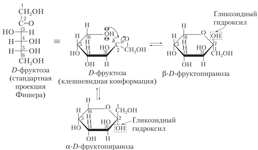
Рис. 13.5. Схема образования пиранозных циклов у D -фруктозы
