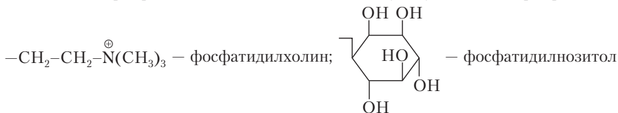
Рис. 17.5. Структурная формула глицерофосфолипидов ( a ) и модель молекулы 1-стеариол-2-олеоил-3-фосфатидилхолина ( b ):
