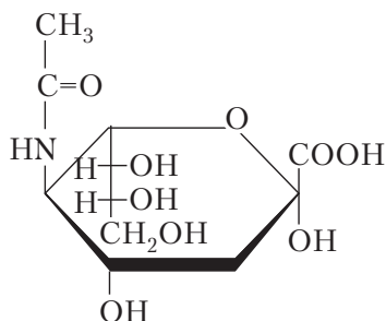
N-ацетилнейраминная кислота
