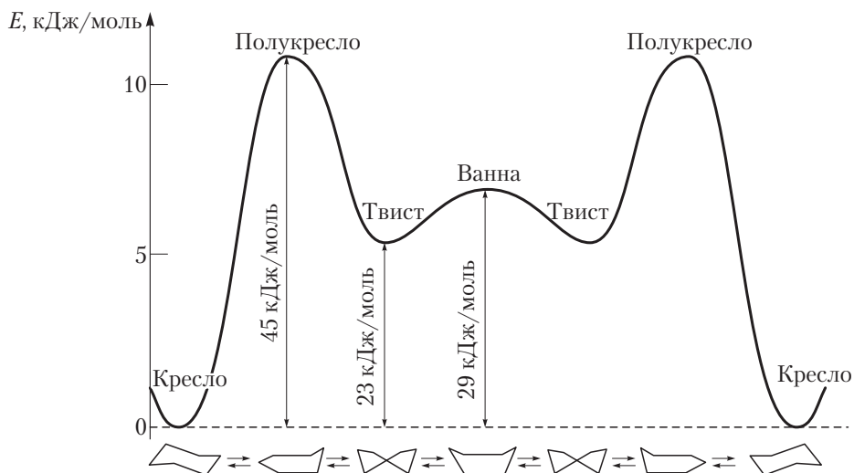
Рис. 3.12. Энергетическая характеристика переходов между конформациями циклогексана
