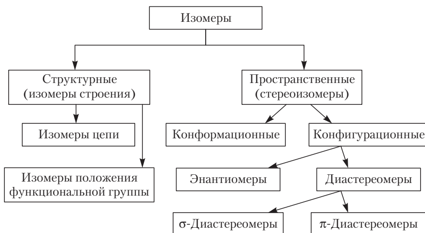
Рис. 3.1. Классификация изомеров
