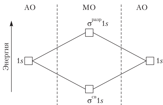
Рис. 2.3. Схема образования связывающей ( \sigma^{\text{св}} ) и разрыхляющей ( \sigma^{\text{разп}} ) МО
