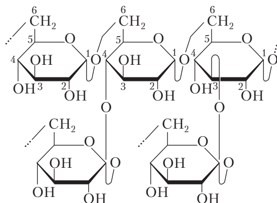
Рис. 13.16. Структура декстрана
