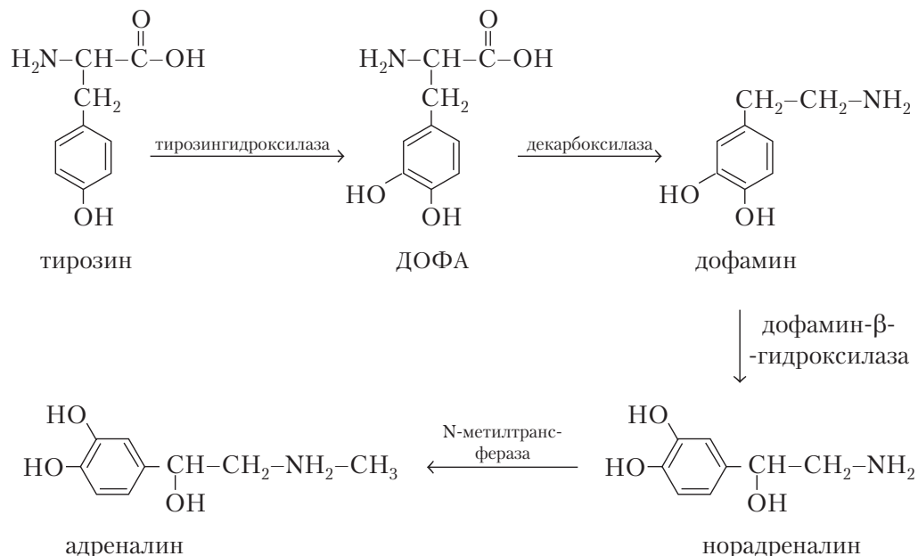
Рис. 14.8. Биосинтез катехоламинов
