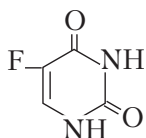
5-фторурацил
