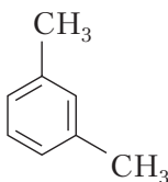
1,3-диметилбензол ( m -ксилол)
