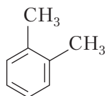
1,2-диметилбензол ( o -ксилол)
