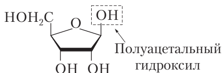
\beta - D -рибофураноза
