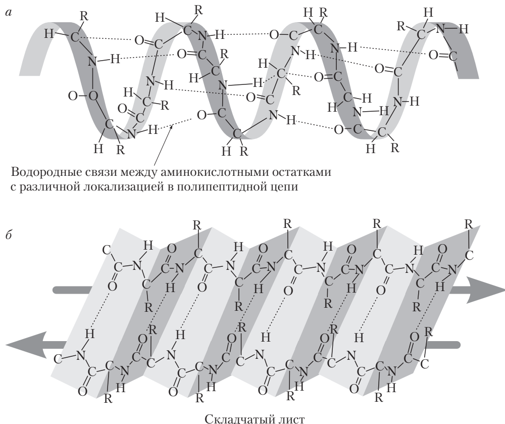
Рис. 15.5. Вторичная структура полипептидной цепи: a — \alpha -спираль; b — \beta -структура
