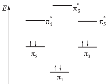
Рис. 2.12. Диаграмма относительных энергий \pi -молекулярных орбиталей бензола: \pi_1, \pi_2, \pi_3 — связывающие МО; \pi_4^*, \pi_5^*, \pi_6^* — разрыхляющие МО
