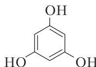
флороглуцин (1,3,5-тригидроксибензол)
