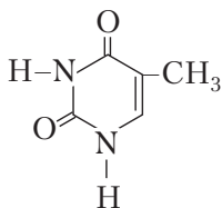
тимин (5-метил-2,4-диокси- пиримидин)
