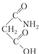
моноамид малоновой кислоты
