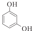
резорцин (1,3-дигидроксибензол)
