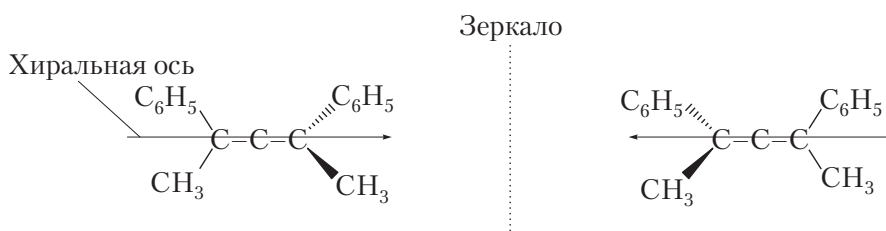
Рис. 3.14. Энантимеры замещенного аллена, имеющего хиральную ось
