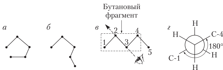
Рис. 3.9. Конформации открытой углеродной цепи: а — клешневидная; б — нерегулярная; в — зигзагообразная; з — заторможенная конформация бутанового фрагмента
