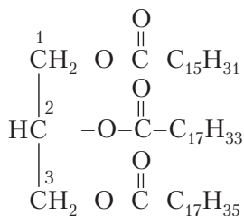
1-пальмитоил-2-олеоил-3-стеароилглицерол
