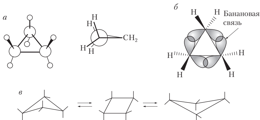
Рис. 3.10. Малые циклы: a — циклопропан; б — «банановая» связь в циклопропане; в — складчатые конформации циклобутана
