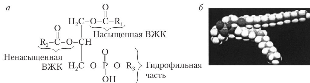
Рис. 17.5. Структурная формула глицерофосфолипидов ( a ) и модель молекулы 1-стеариол-2-олеоил-3-фосфатидилхолина ( b ):
