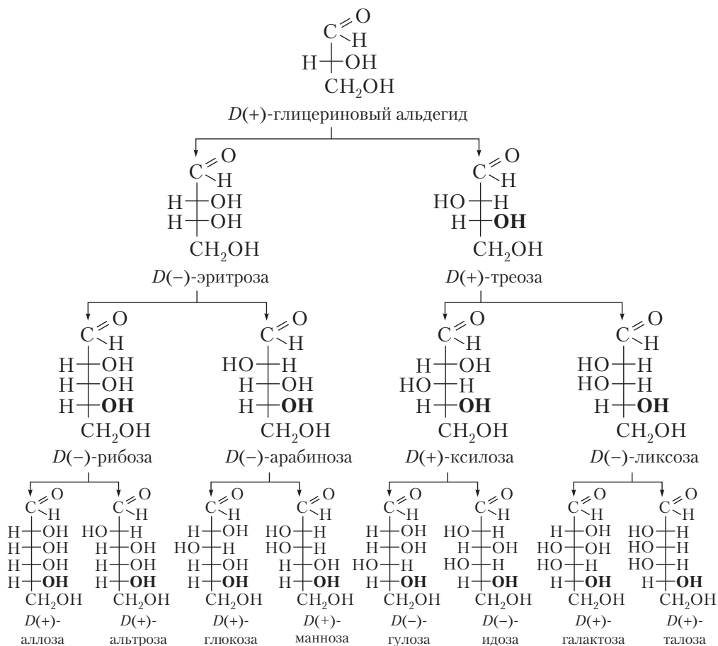
Рис. 13.1. Семейство D-альдоз
