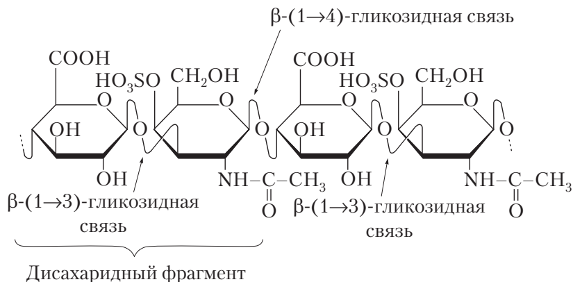
Рис. 13.18. Структура хондроитин-4-сульфата
