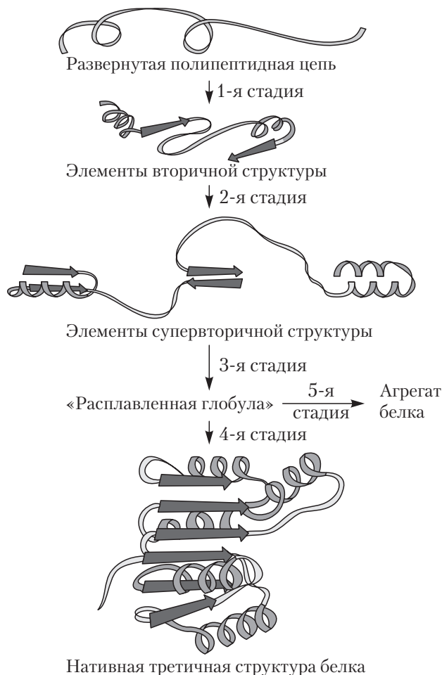
Рис. 15.11. Схема последовательного (постадийного) формирования нативной третичной структуры белка из развернутой вновь синтезированной полипептидной цепи
