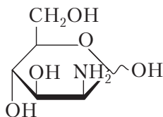
D -маннозамин (2-амино-2-дезоксид- D -маннопираноза)
