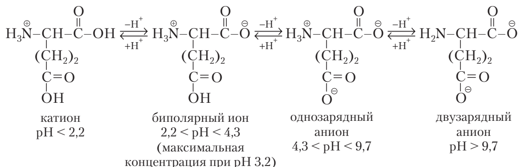
Рис. 14.6. Ионные формы глутаминовой кислоты при разных значениях pH раствора
