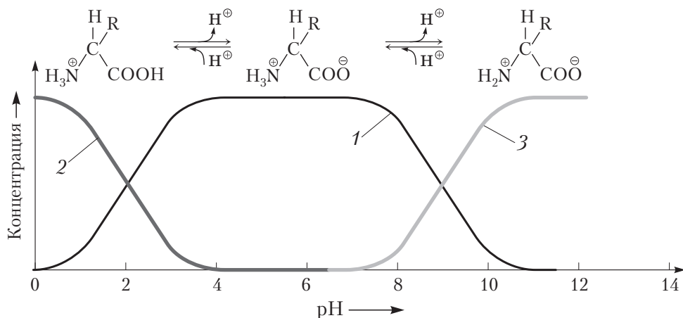
Рис. 14.3. Изменение концентрации равновесных форм ионов в растворе аминокислот в зависимости от рН среды:
