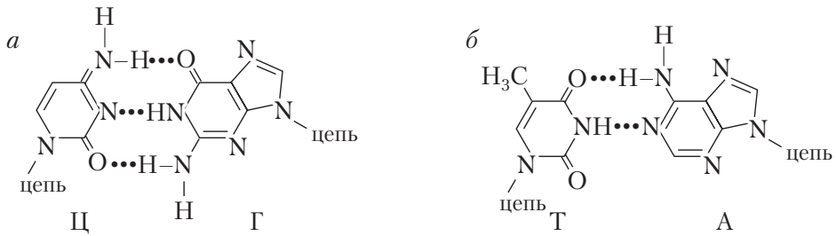
Рис. 16.9. Комплементарные пары азотистых оснований: а – пара ЦГ; б – пара АТ
