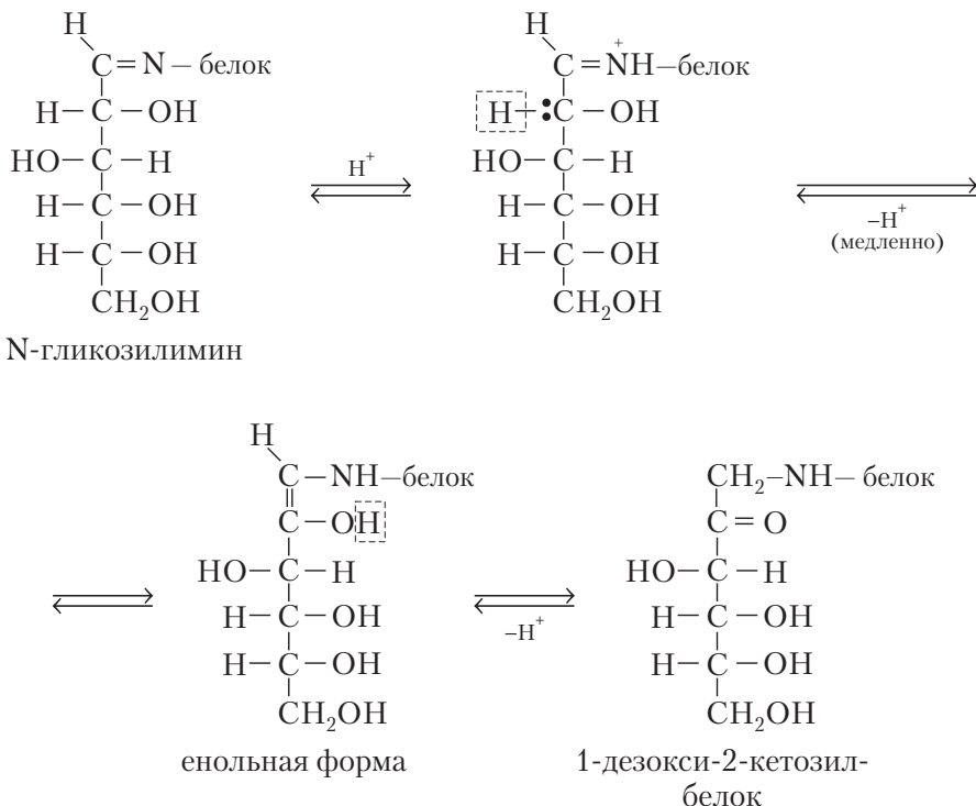
Рис. 13.11. Перегруппировка Амадори
