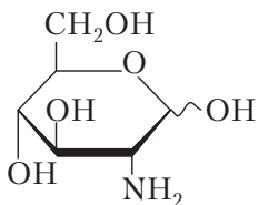
D -глюкозамин (2-амино-2-дезоксид- D -глюкопираноза)
