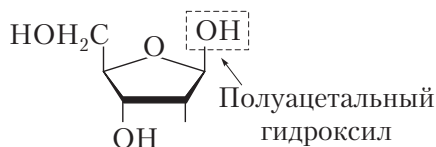
\beta - D -дезоксирибофураноза
