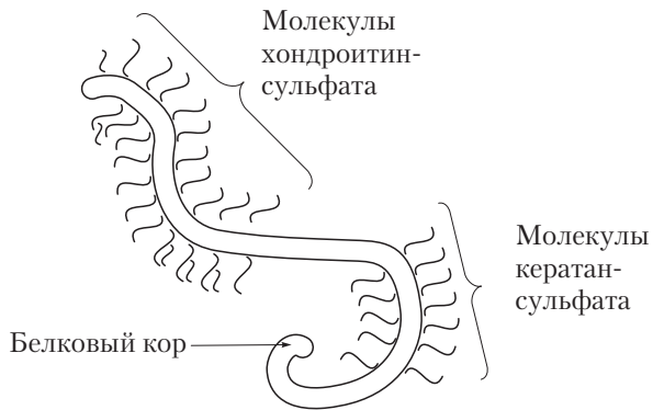
Рис. 13.23. Протеогликановая субъединица
