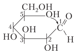
D -глюкоза
