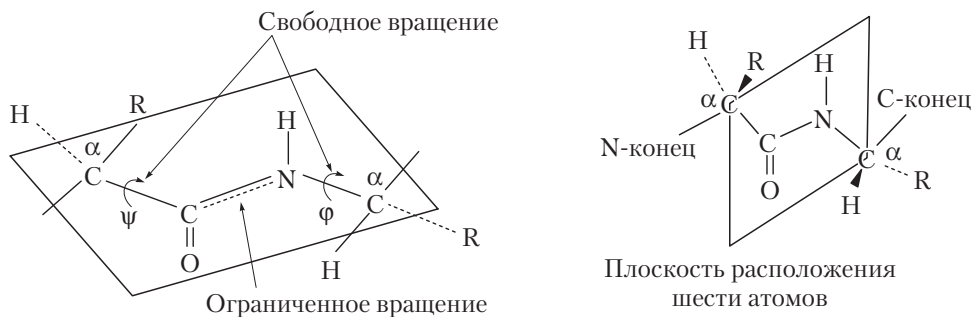
Рис. 15.1. Плоскостное расположение пептидной связи –CO–NH– и \alpha -атомов углерода аминокислотных остатков: \phi , \psi — углы поворота вокруг связей соответственно C–N и C–C
