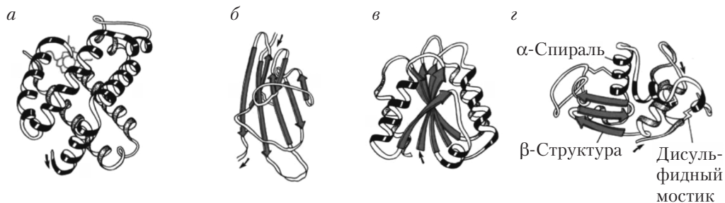
Рис. 15.9. Представители классов белков, разных по характеру тройной структуры: a — \alpha/\alpha -белки — \beta -субъединица гемоглобина; b — \beta/\beta -белки — константный домен иммуноглобулина; v — \alpha/\beta -белки — флаводоксин; z — \alpha+\beta -белки — лизоцим куриного яйца
