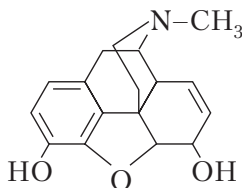
морфин
