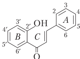
халконы
