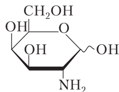
D -галактозамин (2-амино-2-дезоксид- D -галактопираноза)
