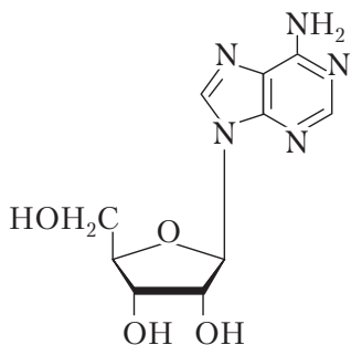
аденозин
