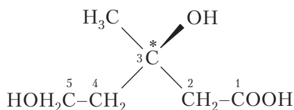
(R)3-метил-3,5-дигидроксипентановая кислота
