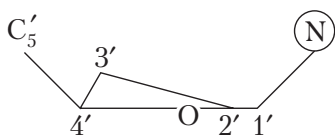
конформация конверта ( E )
