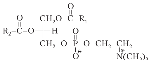
фосфатидилхолин
