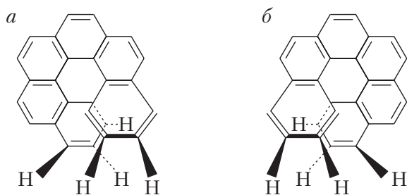
Рис. 3.15. Энантиомеры гексагелицена: a – P -гексагелицен; б – M -гексагелицен
