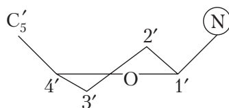
твист -конформация ( T )
