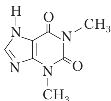
теofilлин (1,3-диметилксантин)
