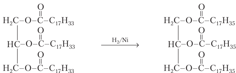
1, 2, 3-триолеилглицерол
