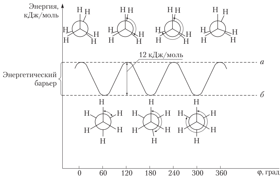
Рис. 3.6. Потенциальная энергия конформаций этана:
