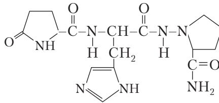
тиреолиберин
