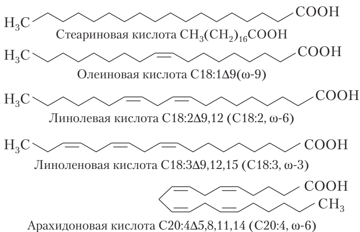
Рис. 17.1. Структура углеводородных цепей некоторых высших жирных кислот (обозначение Cn:1(2,3,4)\Delta m указывает, что ненасыщенная кислота содержит n атомов углерода и одну (2–4) двойную связь у m -го атома углерода, считая первым атомом углерода карбоксильной группы)
