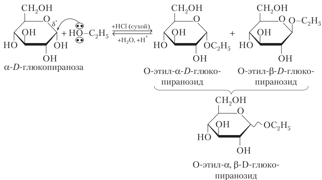
Рис. 13.9. Схема образования O-гликозидов
