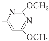
сульфадиметоксин
