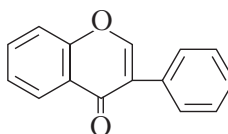
изофлавоны
