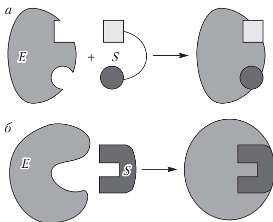
Рис. 3.16. Модели избирательного взаимодействия на молекулярном уровне: a — модель «ключ — замок» Фишера; б — «рука — перчатка» Кошленда
