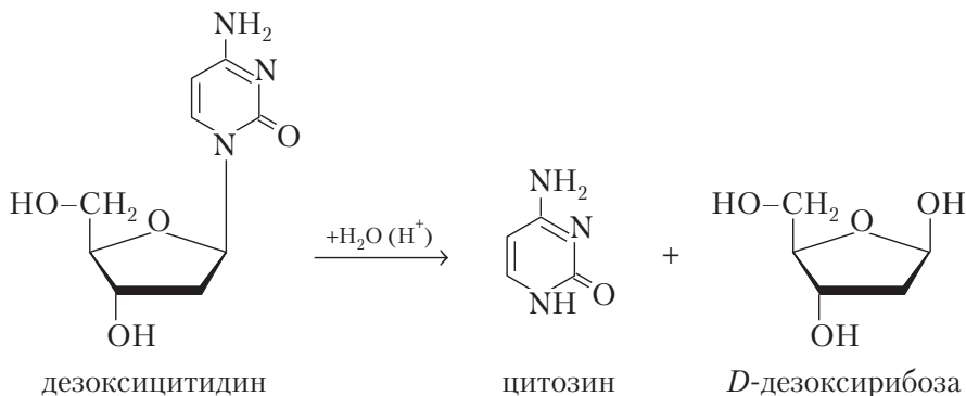
дезоксцитидин
