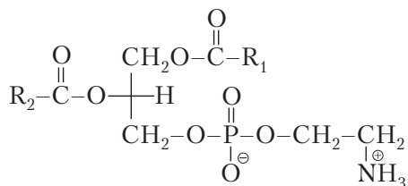
фосфатидилэтаноламин
