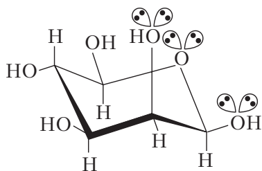
\beta - D -маннопираноза (неустойчивая конформация)
