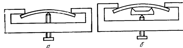
Рис. 12 Схема нагруженных образцов а — сосредоточенной силой, б — чистый изгиб
