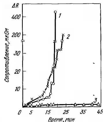
Рис. 10. Изменение омического сопротивления образцов стали 30ХГСНА при коррозии под напряжением, \text{MN/m}^2 ( \text{kgf/mm}^2 ): 1—1110 (111); 2—1650 (165); 3—без напряжения
