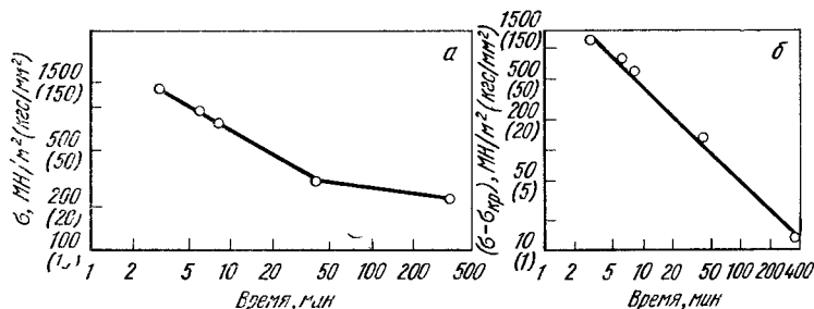
Рис. 16 Кривая коррозионного растрескивания стали 30XГСНА в 20% \text{H}_2\text{SO}_4 + \text{NaCl} (30 кг/м 2 ) в координатах а — \lg \sigma - \lg \tau ; б — \lg (\sigma - \sigma_{\text{кр}}) - \lg \tau
