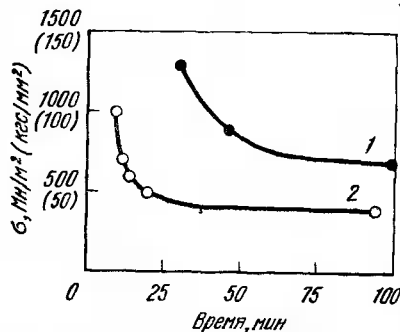
Рис. 42. Влияние молибдена на коррозионное растрескивание стали: 1 — без Mo; 2 — 0,22% Mo
