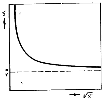
Рис. 54 Кривая водородного растрескивания
