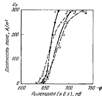
Рис. 68. Влияние количества тиомочевина и pH на катодную поляризацию:
