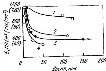
Рис. 38. Кривые коррозионного растрескивания стали с различным содержанием хрома, %: 1 — 0, 2 — 0,56; 3 — 2,48, 4 — 4,3
