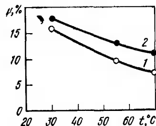
Рис 61 Влияние температуры электролита на пластичность хромированной стали 30ХГСНА при D_k \text{ А/м}^2 1 — 5000, 2 — 7500
