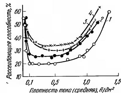
Рис 67 Влияние плотности тока на рассеивающую способность хлористоаммонийного электролита с различным содержанием тиомочевины, \text{кг}/\text{м}^3
