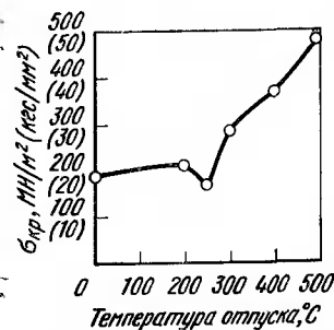
Рис. 46. Влияние температуры отпуска на коррозионное растрескивание стали 30ХГСНА в 20%-ном растворе \text{H}_2\text{SO}_4 + \text{NaCl} (30 кг/м³)
