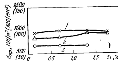
Рис. 41. Влияние кремния на коррозионное растрескивание стали после отпуска при температуре, ^\circ\text{C} : 1 — 350; 2 — 300; 3 — 200
