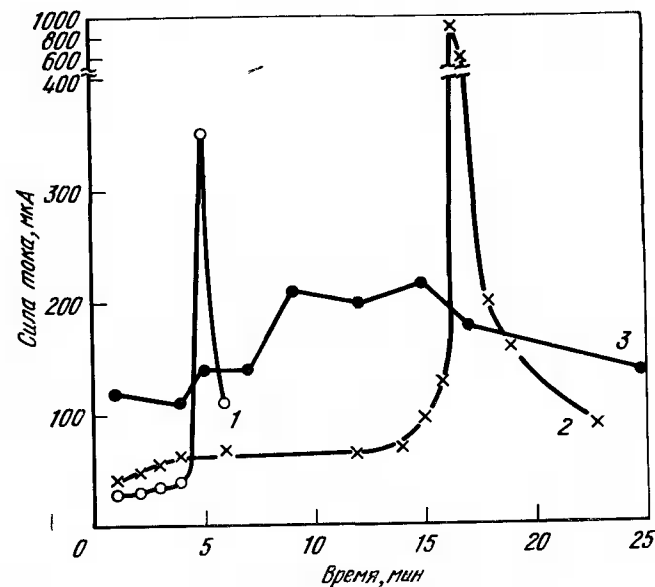
Рис. 13. Влияние состава среды на силу тока пары Fe—Fe (напряженное) стали ВКС-1 1 — 20% \text{H}_2\text{SO}_4 + \text{NaCl} ( 30 \text{ кг/м}^3 ), 2 — 20% ная \text{H}_2\text{SO}_4 ; 3 — (\text{NH}_4)_2\text{S}_2\text{O}_8 ( 100 \text{ кг/м}^3 )
