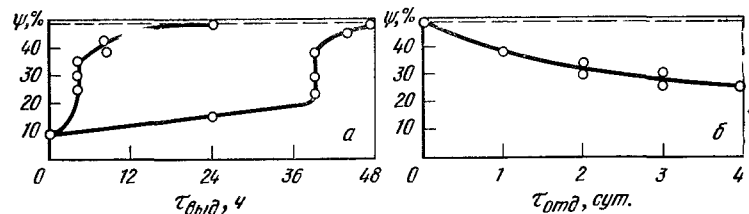
Рис 72 Влияние времени заневоливания ( \tau_{выд} ) (а) и отдыха ( \tau_{отд} ) (б) на пластичность кадмированной стали ( \psi )
