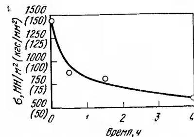
Рис. 63 Влияние растягивающих напряжений при хромировании на время до растрескивания стали 30ХГСА
