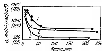
Рис. 39. Кривые коррозионного растрескивания стали с различным содержанием марганца, % (отпуск при 200°С): 1 — 0,68, 2 — 1,57; 3 — 1,88
