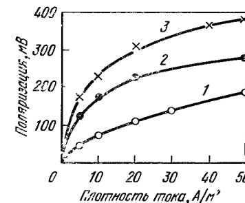
Рис. 23 Катодная поляризация стали 30ХГСНА
