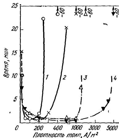
Рис. 57. Влияние плотности тока и концентрации серной кислоты на время до растрескивания стали 40ХГСА: 1 — 0,05 н; 2 — 0,1; 3 — 1,0; 4 — 3,0
