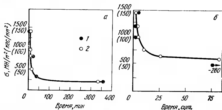
Рис. 15 кривые коррозионного растрескивания сталей в разных средах а — в 20% ной H_2SO_4 + NaCl (30 кг/м³) [1 — экспериментальные значения; 2 — расчетные из уравнения ( \sigma = 214 ) \tau = 4360 МН/м²·мин (436 кгс/мм²·мин)]; б — в камере 3% NaCl [1 — экспериментальные значения; 2 — расчетные из уравнения ( \sigma = 575 ) \tau = 2050 МН/м²·сутки (205 кгс/мм²·сутки)]
