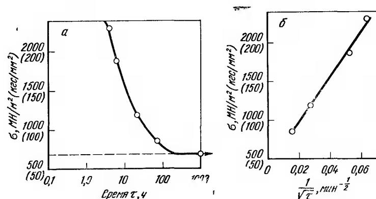
Рис. 69. Кривые статической водородной усталости стали 30ХГСНА, кадмированной в цианистом электролите \sigma - \lg \tau (а) и \sigma - \frac{1}{\sqrt{\tau}} (б)
