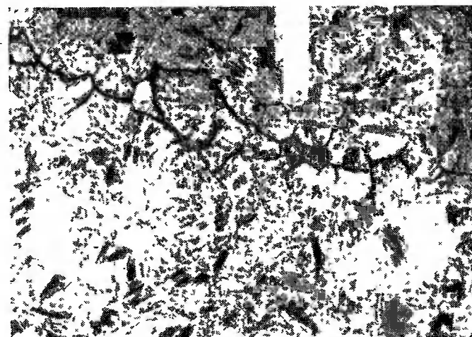
Рис. 27. Трещины, образующиеся при коррозии под напряжением стали 30ХГСНА в растворе едкого натра с нитритом натрия ×500
