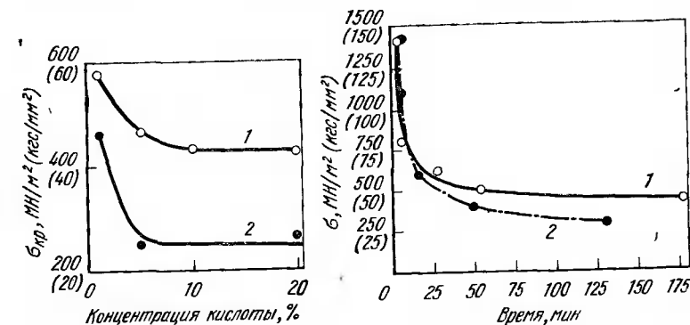
Рис. 18 Влияние концентрации кислот на коррозионное растрескивание стали 30ХГСНА
