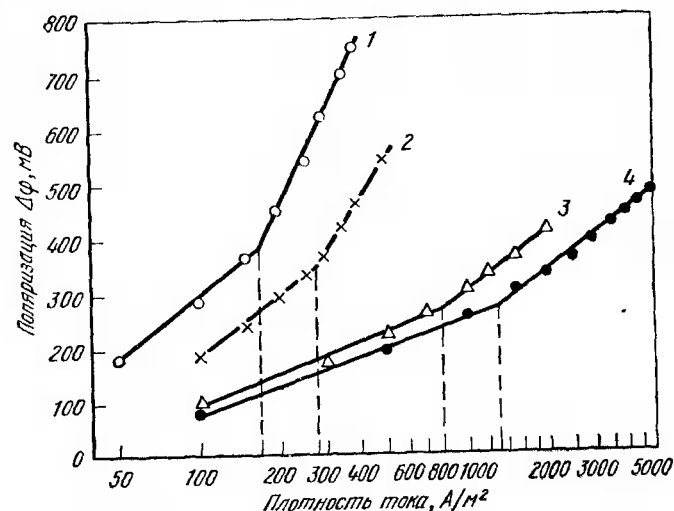
Рис. 58. Зависимость катодной поляризации \Delta\phi стали 40ХГСНА от плотности тока в H_2SO_4 : 1—0,05 н; 2—0,1; 3—1,0, 4—3,0
