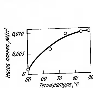
Рис. 74. Влияние температуры фосфатирующего раствора на массу пленки (время обработки 15 мин)
