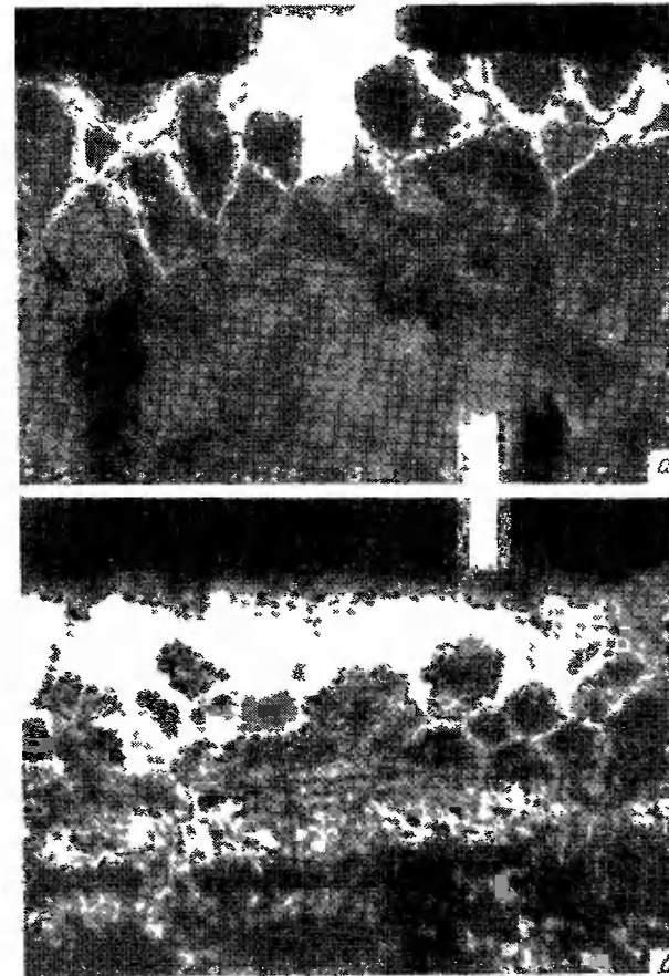
Рис. 50 Влияние среды нагрева под закалку на характер обезуглероживания стали а — нагрев в соляной ванне, б — в воздушной печи
