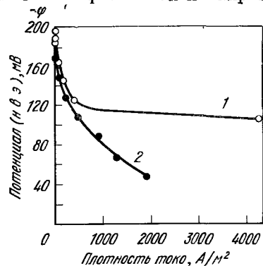
Рис. 3 Влияние растягивающих напряжений на анодную поляризацию стали ВКС-1 1 — напряжение 1000 МН/м² (100 кгс/мм²), 2 — без напряжений
