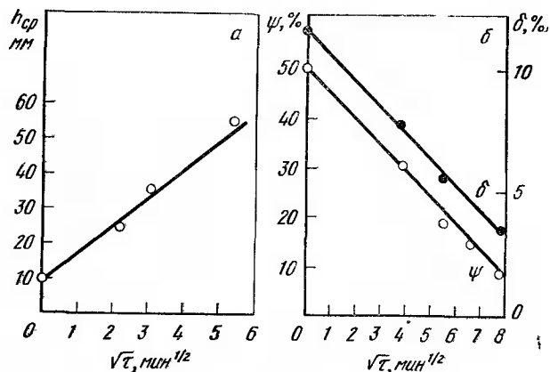
Рис. 52. Зависимость пластичности стали от продолжительности травления в координатах. а — h_{cp} - \sqrt{t} , б — \psi - \sqrt{t} , \delta - \sqrt{t}
