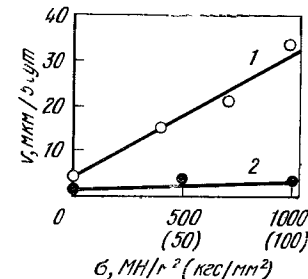
Рис. 7. Влияние растягивающих напряжений на скорость коррозии стали 30ХГСНА. 1 — 3%-ный раствор NaCl + 0,1%-ный H 2 O 2 . 2 — 3%-ный раствор NaCl
