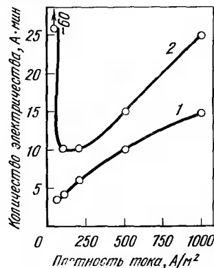
Рис. 65. Влияние плотности тока на количество электричества, необходимого для водородного растрескивания стали 40ХГСНА под напряжением, \text{МН/м}^2 ( \text{кгс/мм}^2 ), при цинковании в цианистом электролите: 1 — 1200 (120), 2 — 1000 (100)
