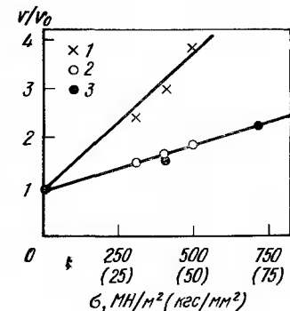
Рис. 6. Влияние растягивающих напряжений на скорость коррозии стали 30ХГСНА ( v — скорость коррозии при данном растягивающем напряжении, v_0 — то же без напряжений) 1 — 20% \text{H}_2\text{SO}_4 + \text{NaCl} (30 \text{кг/м}^3 ) 2 — 20% \text{H}_2\text{SO}_4 . 3 — 3% \text{NaCl} + 0,1% \text{H}_2\text{O}_2
