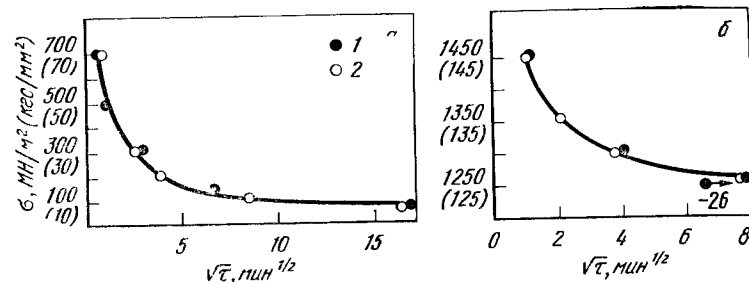
Рис. 55 Кривые водородного растрескивания стали 30ХГСНА а — в 20%-ной H_2SO_4 + NaCl (30 кг/м 3 ), D_K=100 А/м 2 , б — в NaOH (100 кг/м 3 ) + NaCN (10 кг/м 3 ), D_K=150 А/м 2 (1 — экспериментальные значения, 2 — расчетные)
