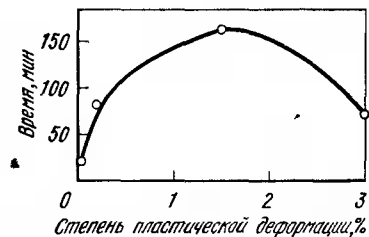
Рис. 31. Влияние пластической деформации на коррозионное растрескивание стали 30ХГСА при напряжении 700 МН/м 2 (70 кгс/мм 2 )
