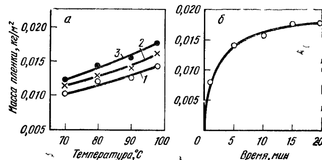
Рис 73 Влияние температуры раствора на массу фосфатной пленки после обработки в течение: 1—5 мин, 2—10, 3—15 (а) и времени обработки на массу фосфатной пленки (б)
