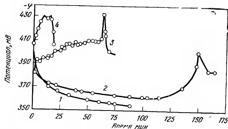
Рис. 2 Влияние растягивающих напряжений [ \text{МН/м}^2 ( \text{кгс/мм}^2 )] на электродный потенциал стали ЭИ643 (по отношению к насыщенному каломельному полуэлементу) 1 — без напряжений, 2 — 975 (97,5); 3 — 1460 (146), 4 — 1800 (180) (расчетные значения)
