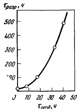
Рис 70. Влияние продолжительности отдыха ( \tau_{отд} ) на время до разрушения ( \tau_{разр} ), кадмированных образцов с надрезом при \sigma = 1700 \text{ МН/м}^2 ( 170 \text{ кгс/мм}^2 )
