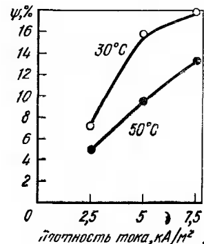
Рис 62 Влияние плотности тока на пластичность хромированной стали 30ХГСНА
