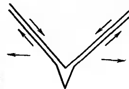
Рис. 33 Возникновение концентратора напряжений по Коттреллу
