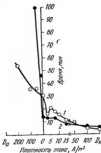
Рис. 21 Влияние катодной и анодной поляризации на коррозионное растрескивание стали ВКС-1 при напряжении 600 \text{ МН/м}^2 ( 60 \text{ кгс/мм}^2 ) в 20%-ной H_2SO_4 (1) и 20%-ной H_2SO_4 + NaCl ( 30 \text{ кг/м}^3 ) (2)
