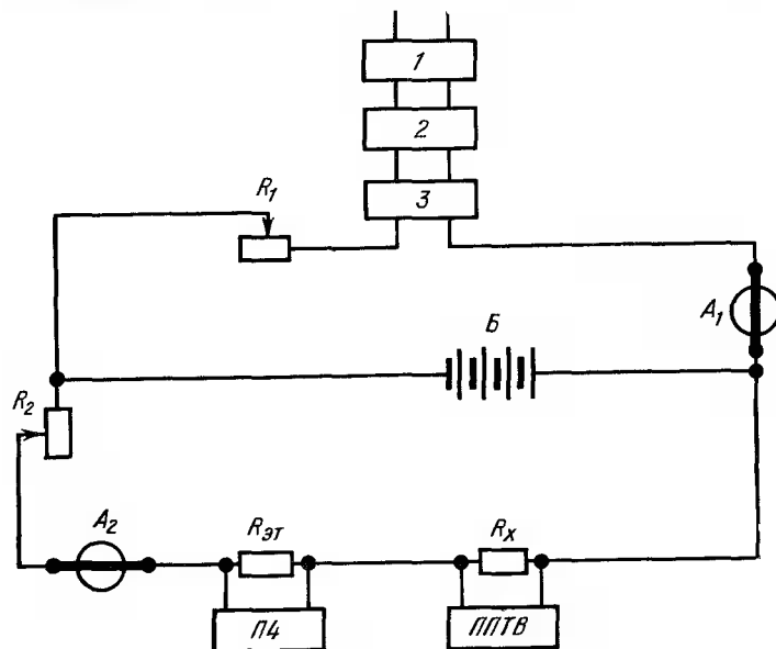
Рис. 8. Установка для измерения сопротивления (схема)
