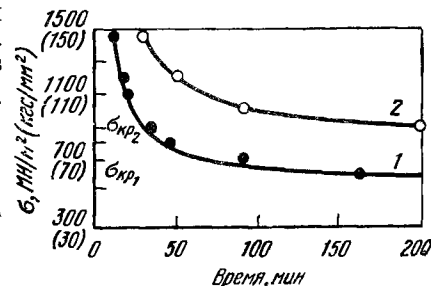
Рис. 44 Влияние раскисления на коррозионное растрескивание стали 30ХГСНА. 1 — без дополнительного раскисления, 2 — раскисление титаном
