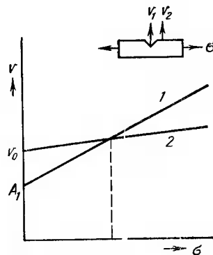
Рис 14 Влияние напряжений на скорость коррозии (схема) 1 — в концентраторе напряжений, 2 — на остальной поверхности
