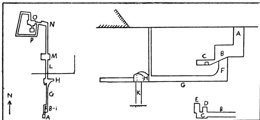
Лабиринт пирамиды Сенусерта II (XIX в. до н. э.)
