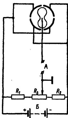
Рис. 15. Схема «квадратного» включения электрометра:
