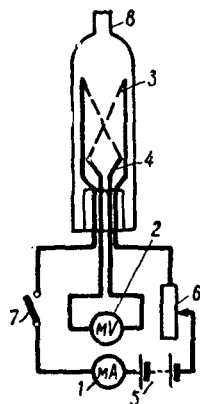
Рис. 70. Схема включения манометрической лампы термопарного вакуупора:
