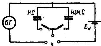
Рис. 101. Схема определения емкости при помощи баллистического гальванометра:
