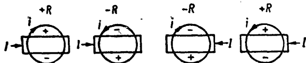
Рис. 116. Иллюстрация правила определения знаков постоянной Холла:
