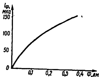
Рис. 103. График световой характеристики селенового фотосопротивления.
