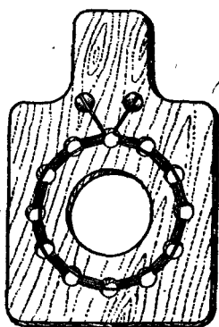
Рис. 40. Пробная катушка.
