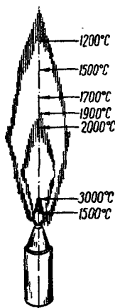
Рис. 60. Распределение температуры в пламени горелки.
