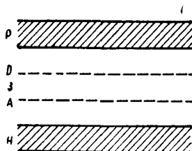
Рис. 91. Зонная диаграмма для полупроводника с примесями: D — дойорные уровни; A — акцепторные уровни.
