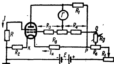
Рис. 16. Вариант мостовой схемы на лампе 1Э1П.
