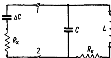
Рис. 30. Эквивалентная схема включения.
