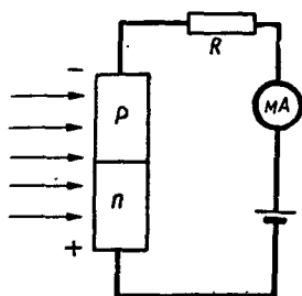
Рис. 139. Фотодиодные включения фотоэлемента.
