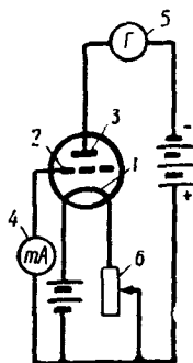
Рис. 71. Схема включения манометрической лампы ионизационного вакуумметра:
