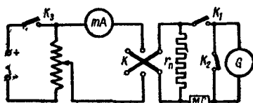
Рис. 8. Схема измерения параметров гальванометра:
