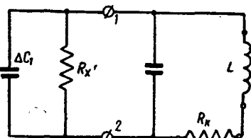
Рис. 31. Эквивалентная схема включения.
