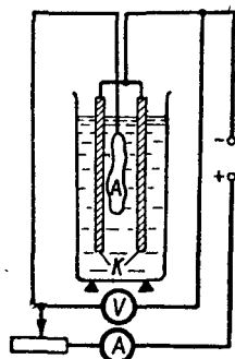
Рис. 57. Схема электрополировки.
