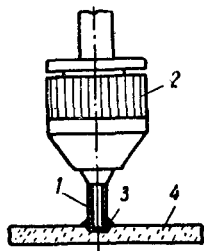
Рис. 58. Сверление отверстий:
