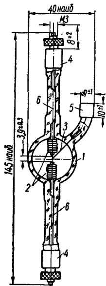
Рис. 44. Ртутная кварцевая лампа.
