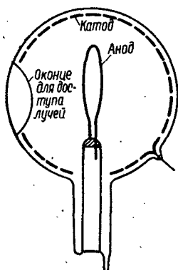
Рис. 50. Принципиальное устройство фотоэлемента с внешним фотоустройством.
