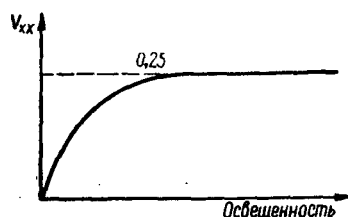
Рис. 135. Зависимость э. д. с. холостого хода от освещенности.
