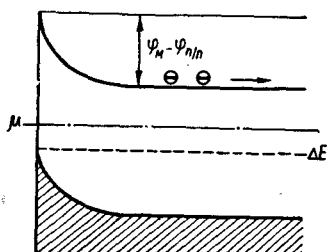
Рис. 134. Зонная диаграмма константы металл—полупроводник.
