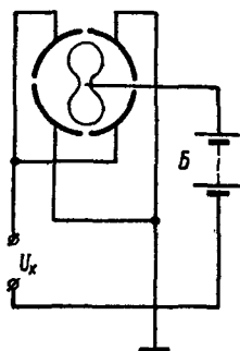
Рис. 14. Схема «бисквитного» включения квадратного электрометра:
