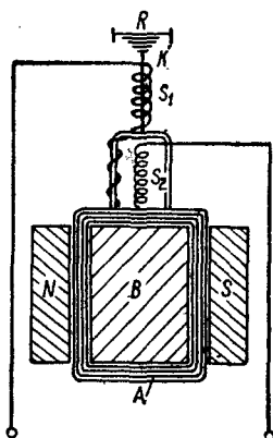
Рис. 41. Эскиз флюксметра.
