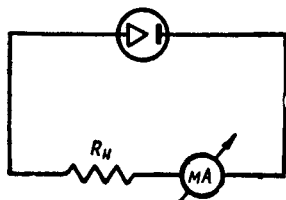
Рис. 136. Схема включения фотоэлемента на внешнее сопротивление. R_n — внешнее сопротивление (нагрузки).
