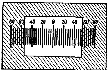
Рис. 3. Шкала вибрационного гальванометра.
